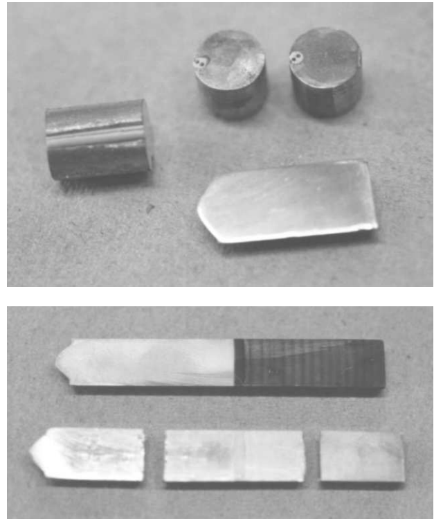
Figura 3: Macrográficas de muestras crecidas bajo distintas condiciones. Se observan los cortes longitudinales y transversales.
