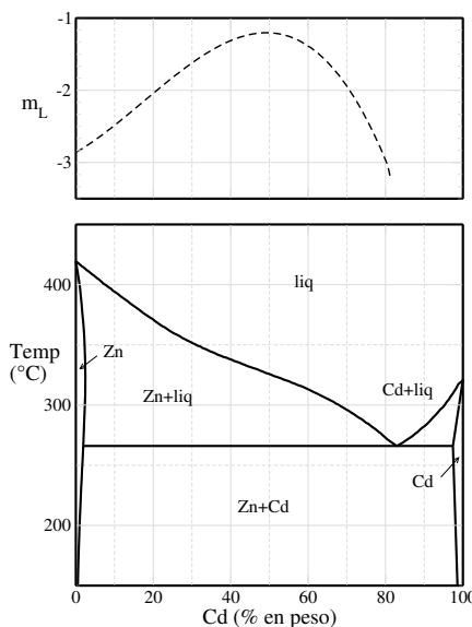
Figura 7: Diagrama de fases del sistema Zn-Cd
