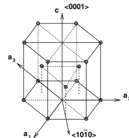
Figura 1: Estructura cristalina apilamiento de la una estructura HCP, donde se muestra esquemáticamente las direcciones preferenciales de crecimiento \langle 0001 \rangle y \langle 10\bar{1}0 \rangle
