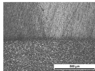
Figura 4: Interfaz plana templada. \text{Zn-0.01\%Cd} . Se observa que el frente templado permite la formación de dos granos diferentes.
